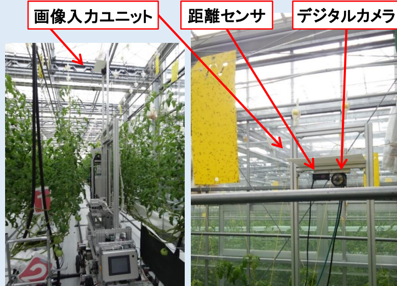
ロボットによる自動撮影
